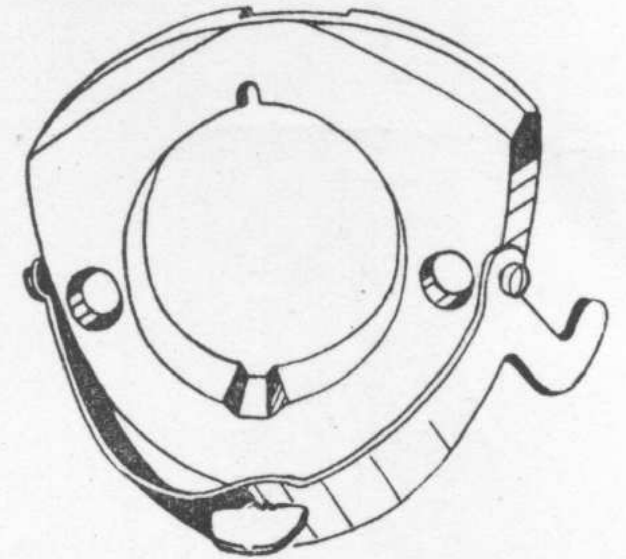
Greiferbahndeckel
